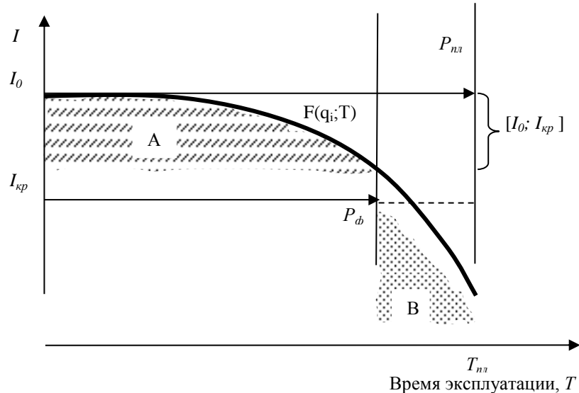
Рис. 2. Взаимосвязь уровня качества продукции и ее ресурса (случай несоответствия ресурса фактического его плановому значению)
