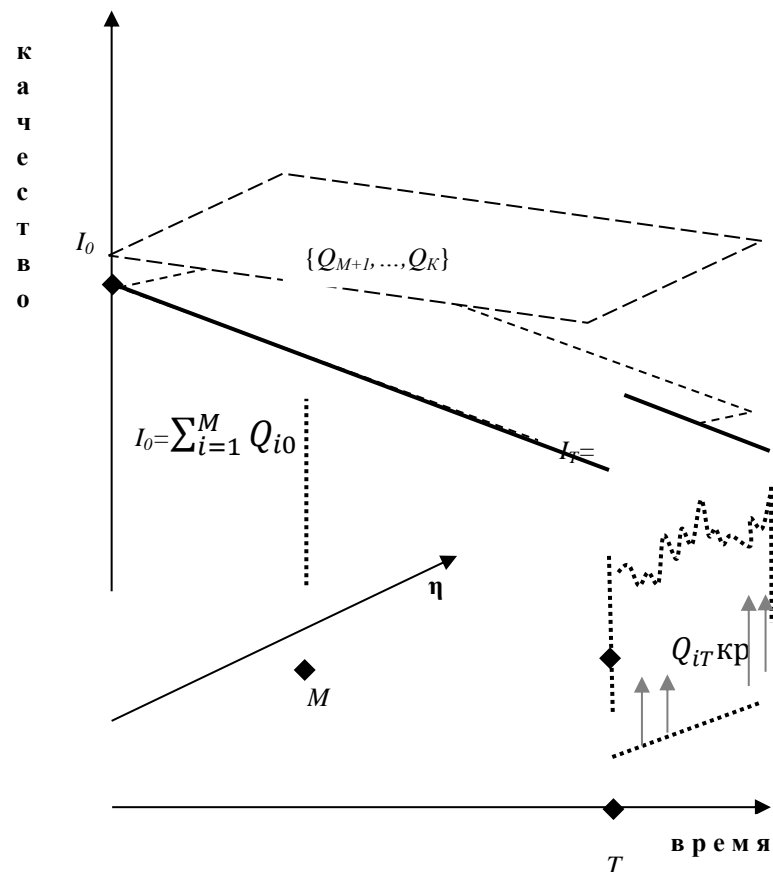
Рис. 1. Модель изменения качества продукции в процессе эксплуатации
