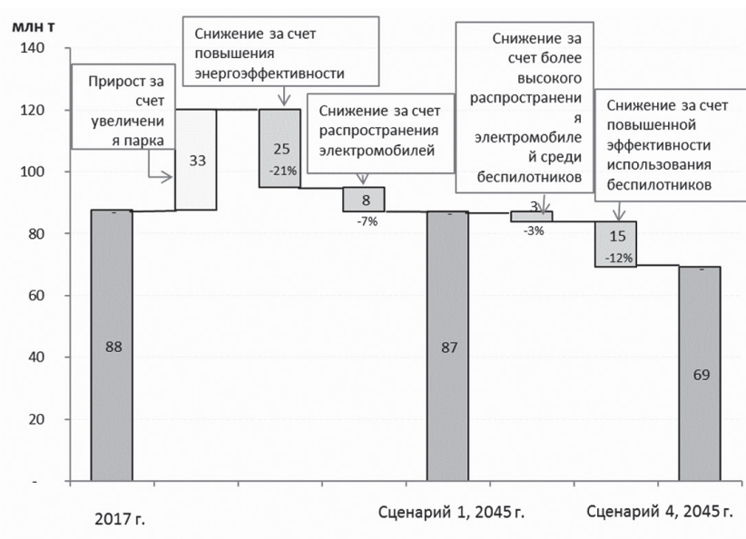
Рис. 1. Вклад отдельных факторов в объемы выбросов диоксида углерода на легковом автотранспорте в России в сценариях 1 и сценарии 4, млн т
