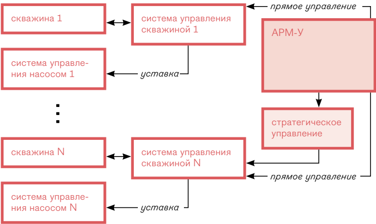
рис. 01 —> Общая схема управления интеллектуальным месторождением
