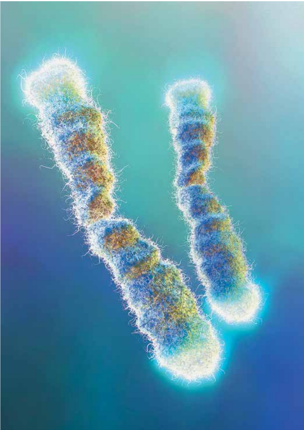
ДНК-полимераза не способна копировать ДНК полностью, с самого начала до самого конца, поэтому теломеры, концевые участки хромосом, при каждой репликации ДНК, то есть при каждом делении клетки, сокращаются. В принципе существует фермент теломераза, который достраивает ДНК до прежней длины, но в большинстве клеток он заблокирован
