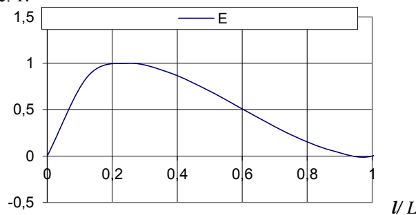
Рис. 1. График распределения энергии по длине флуктуаций
