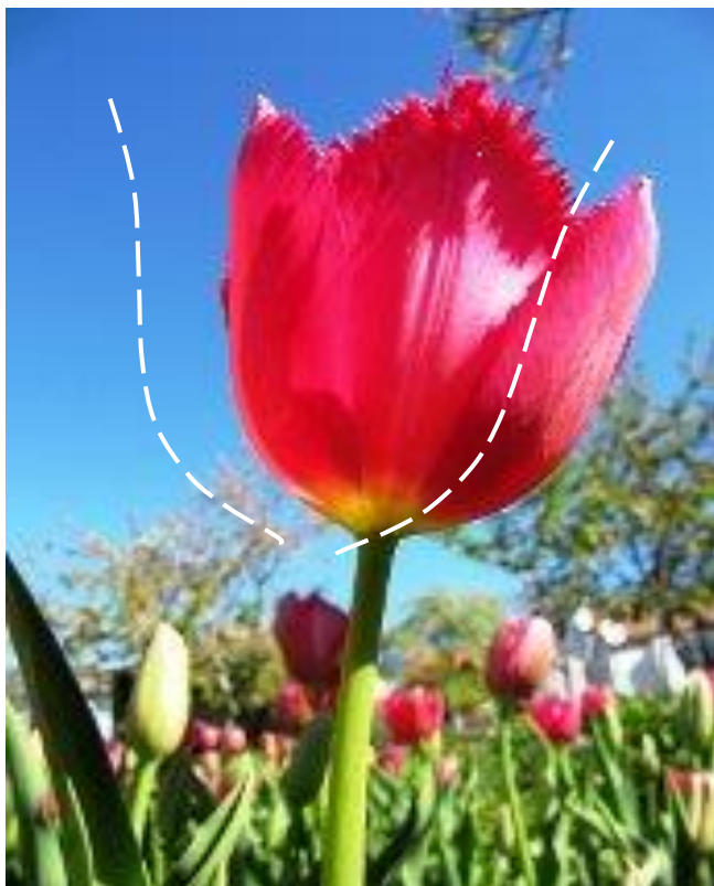
Рис. 15. Сравнение формы цветка тюльпана с теоретической кривой распределения энергии турбулентности по его длине
