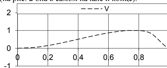
Рис. 3. Теоретический график распределения энергии по длине волны
