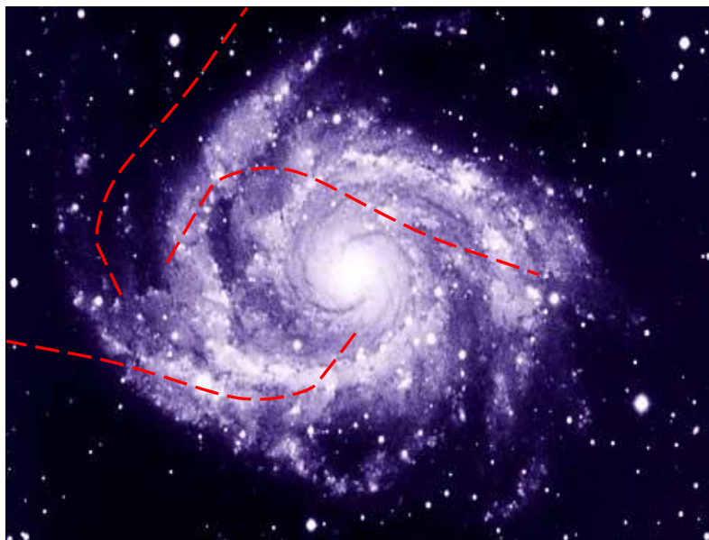
Рис. 5. Фотография галактики 1355607039_6777 в сопоставлении с расчетными волнами распределения в ней энергии турбулентности
