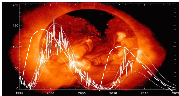
Рис. 6. Солнечная активность (сплошная линия) последних десятилетий в сопоставлении с 11—12-летними волнами энергии турбулентных колебаний большой среды (штриховые линии)
