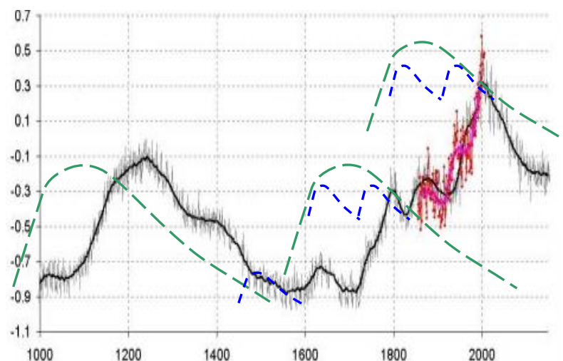
Рис. 12. Вариации температуры на Земле, по данным University of East Anglia, UEA, отдел климатических исследований [4] в сопоставлении с турбулентными волнами активности природной среды 560 и 140-летней продолжительности (штриховые линии)
