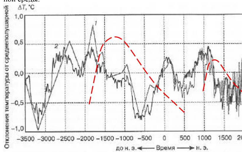
Рис. 13. Волны климатических изменений, по данным А. Никонова [5], сопоставление с 2800-летними и 1120-летними обертонами 140-летней глобальной волны
